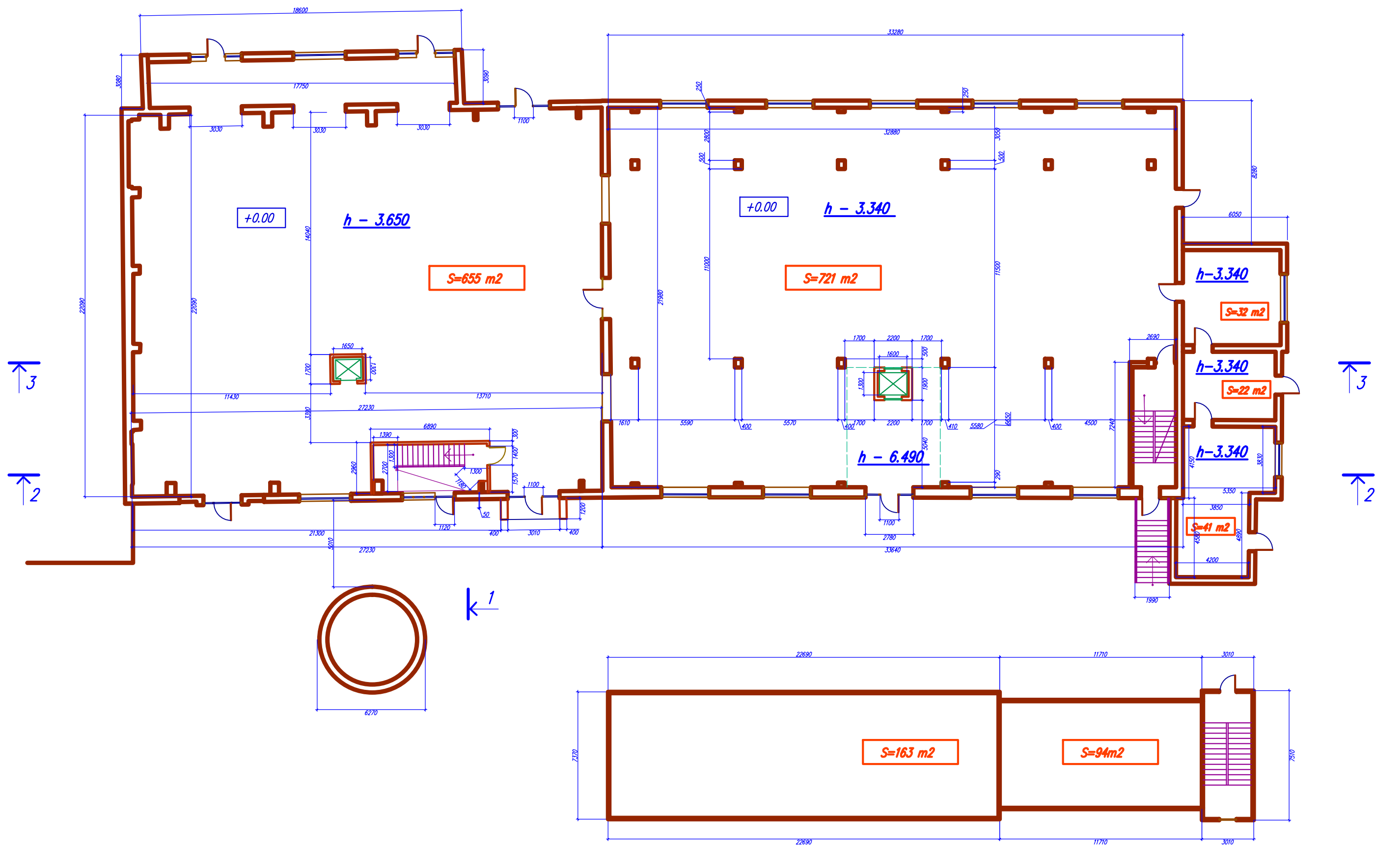
План 1-этажа
