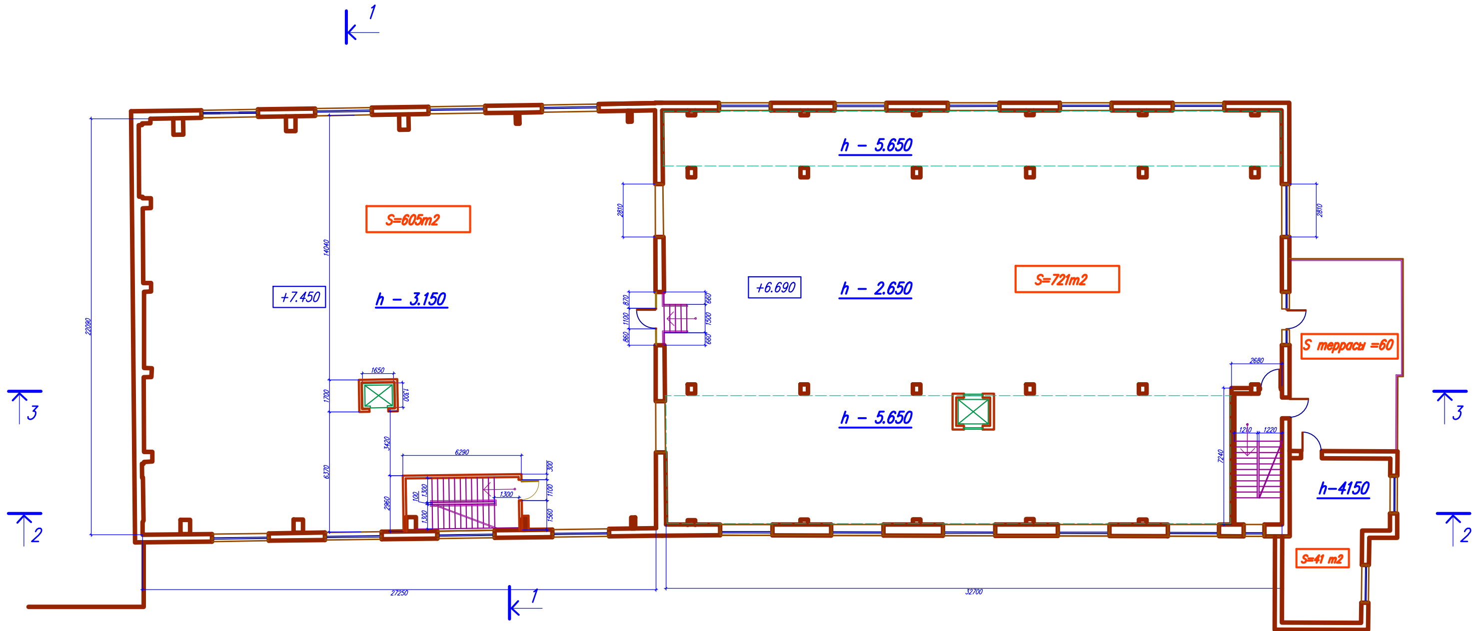
План 3-этажа
